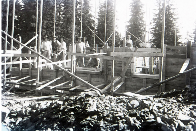
Schalung und Beton
